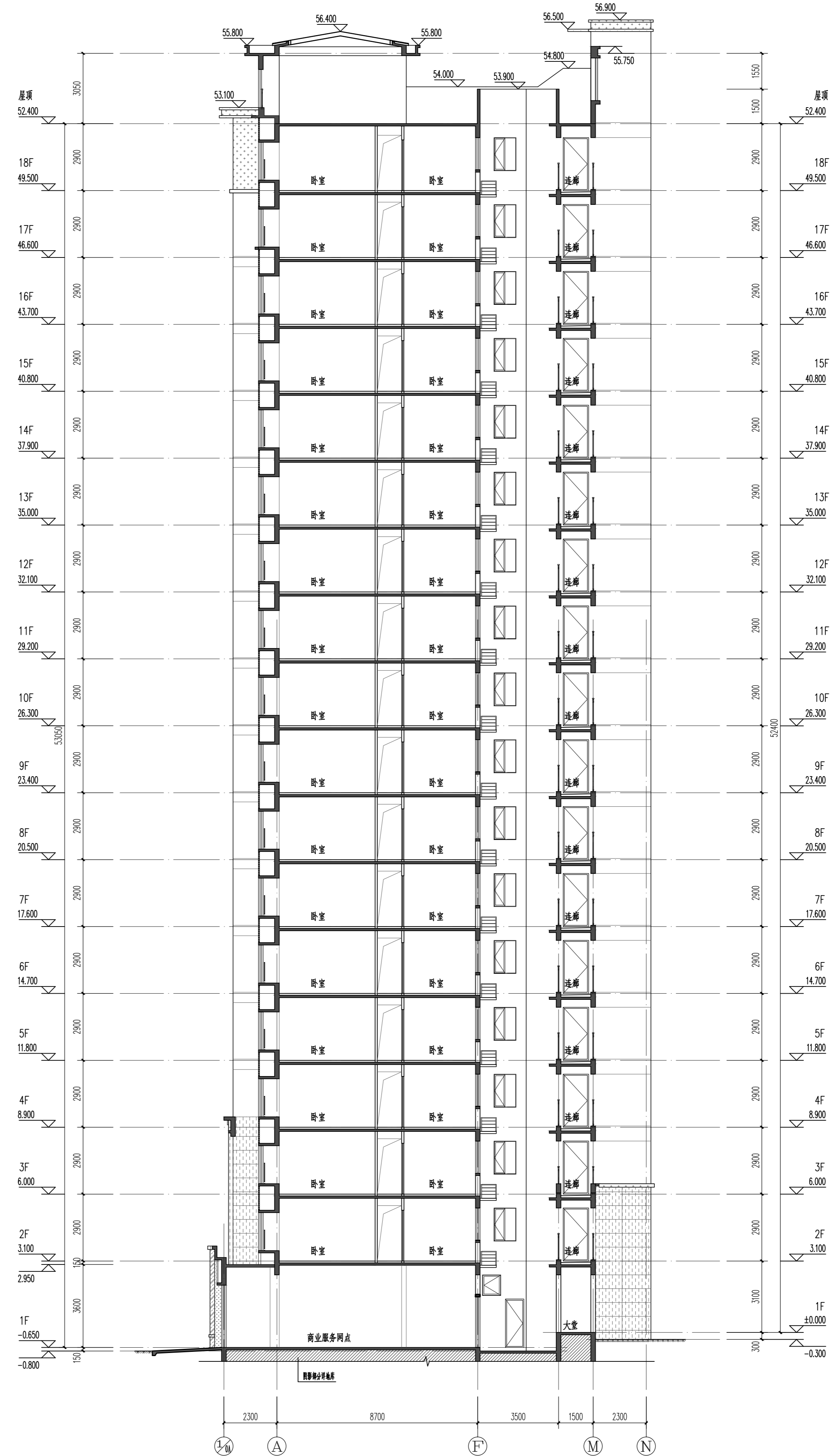
2-2剖面图 1:100
